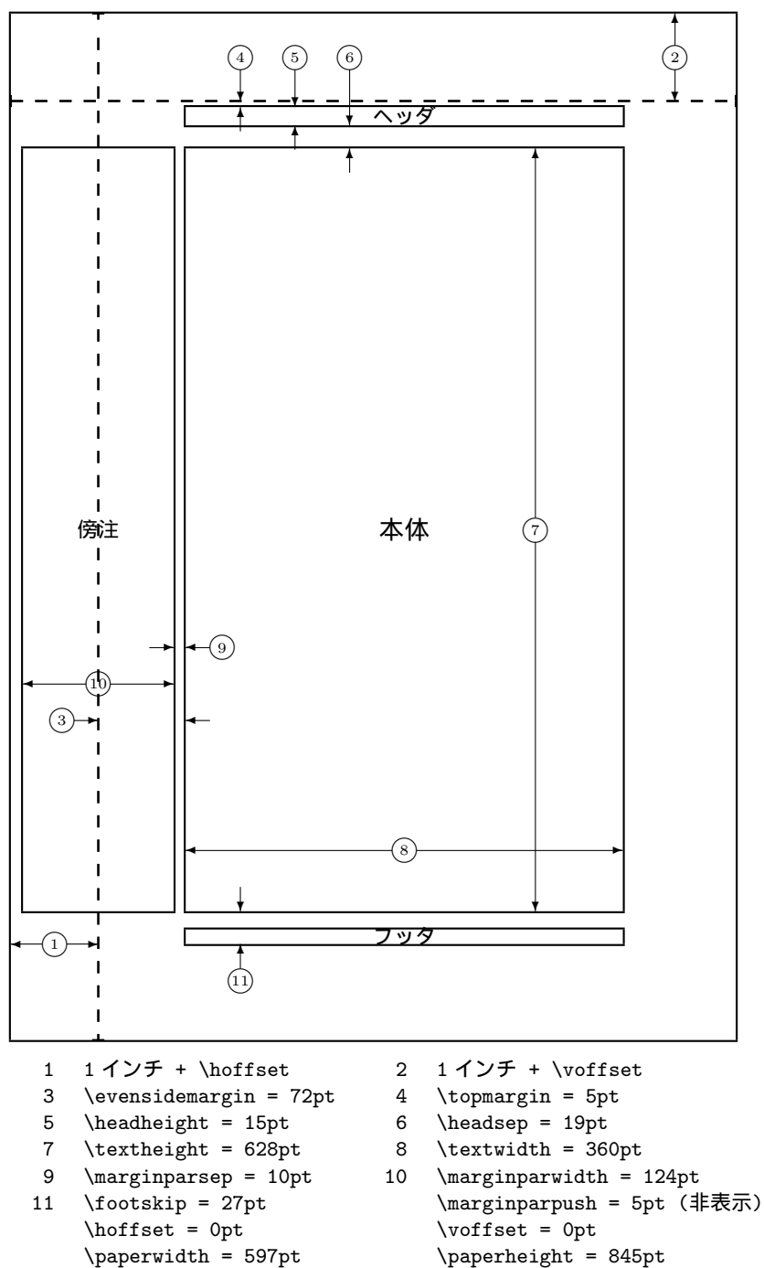
図 5.2: ページレイアウトパラメータ
